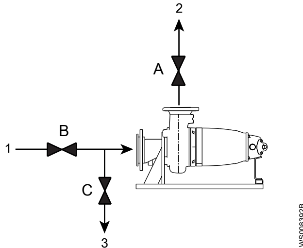
Afbeelding 19: Kleppen A-D voor T-installatie (generieke pomp weergegeven)
