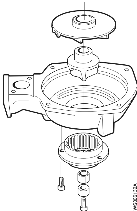
Afbeelding 18: M-waaier
