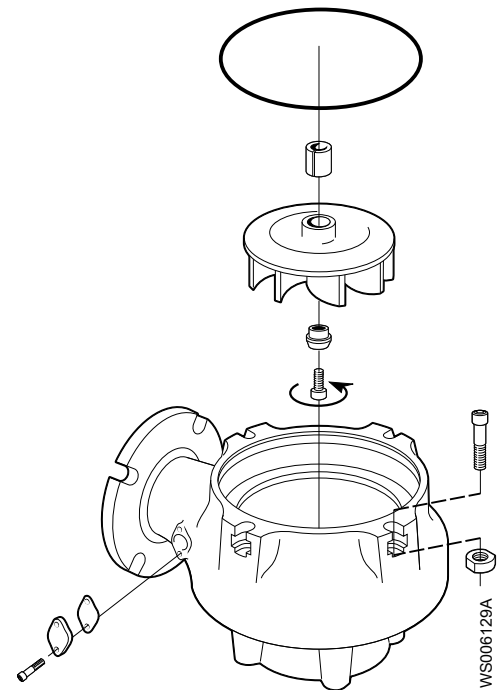
Afbeelding 14: D-waaier
