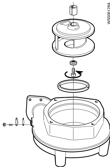
Afbeelding 13: C-waaier
