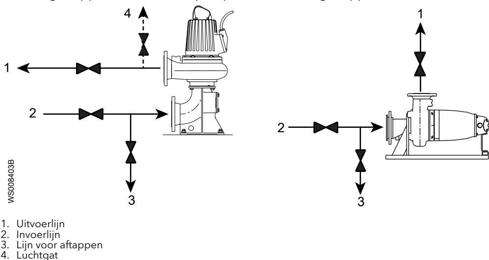
Afbeelding 6: T-, Z-installatie-afsluiting en luchtafsluitventielen (generieke pompen weergegeven)
