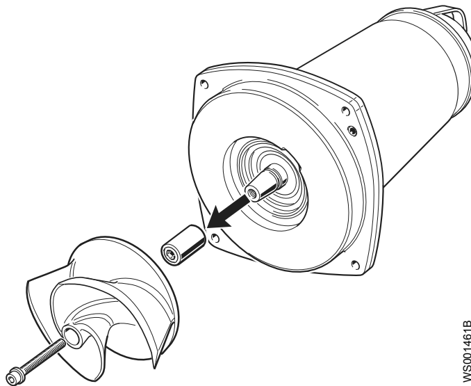
Afbeelding 27: De waaieren en de conische mof verwijderen. Generieke aandrijving afgebeeld.
