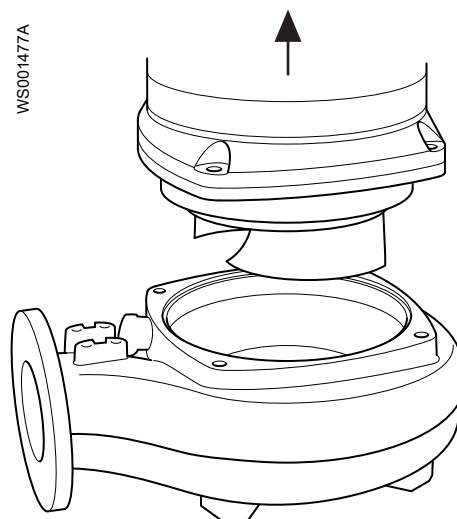
Afbeelding 25: De aandrijving verwijderen. Generieke aandrijving afgebeeld.
