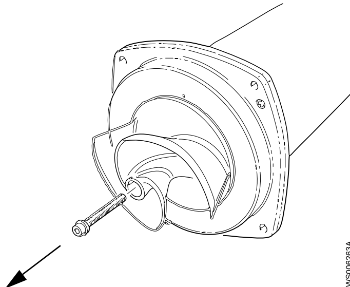
Afbeelding 26: De waaierschroef verwijderen. Generieke aandrijving afgebeeld.
