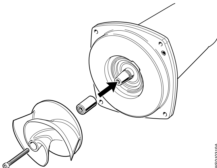
Afbeelding 28: De mof en de waaier op de as plaatsen. Generieke aandrijving afgebeeld.
