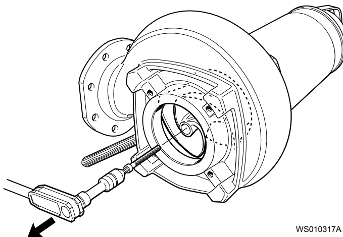
Afbeelding 30: De waaierschroef verwijderen. Generieke aandrijving afgebeeld.
