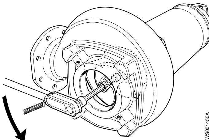
Afbeelding 22: De stelschroef linksom draaien. Generieke aandrijving afgebeeld. e) Draai de waaierschroef handvast om te voorkomen dat deze eraf valt.
