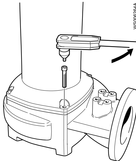
Afbeelding 24: De pomphuis Schroeven verwijderen. Generieke aandrijving afgebeeld.
