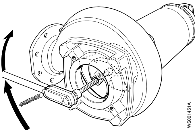
Afbeelding 31: De waaier afstellen. Generieke aandrijving afgebeeld.
