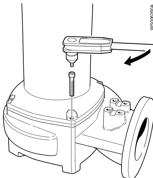
Afbeelding 29: Het pomphuis plaatsen. Generieke aandrijving afgebeeld.
