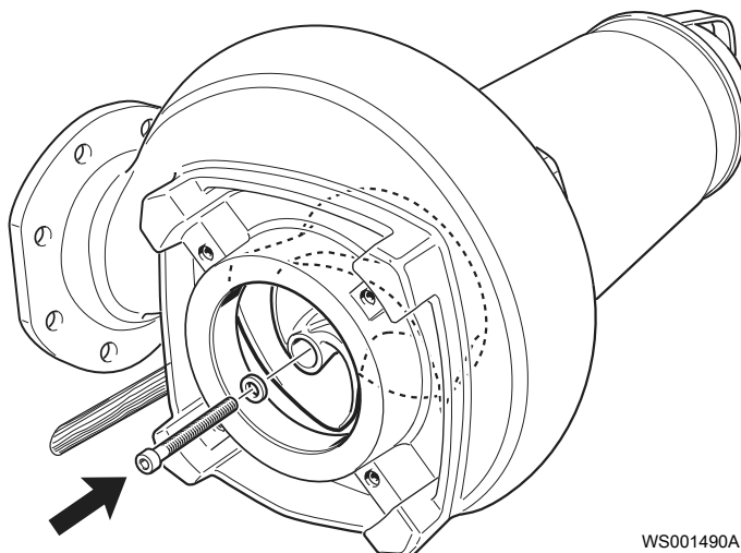
Afbeelding 23: Draai de waaierschroef handvast. Generieke aandrijving afgebeeld. f) Verwijder de staaf. 3. Til de pomp op. 4. Verwijder de aandrijving uit de pompbehuizing: a) Verwijder de schroeven van de pompbehuizing.
