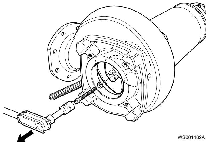
Afbeelding 21: De waaierschroef verwijderen. Generieke aandrijving afgebeeld. d) Draai de stelschroef tegen de klok in tot de waaier los komt van de as.
