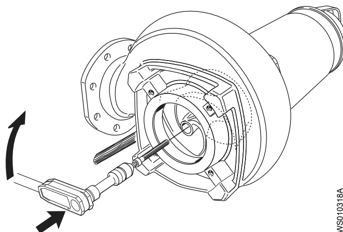
Afbeelding 32: De waaier vastmaken. Generieke aandrijving afgebeeld.
