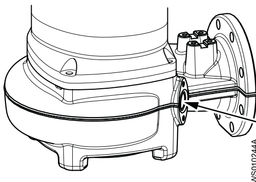
Afbeelding 20: Gat om de stang in te steken. Generieke aandrijving afgebeeld.
