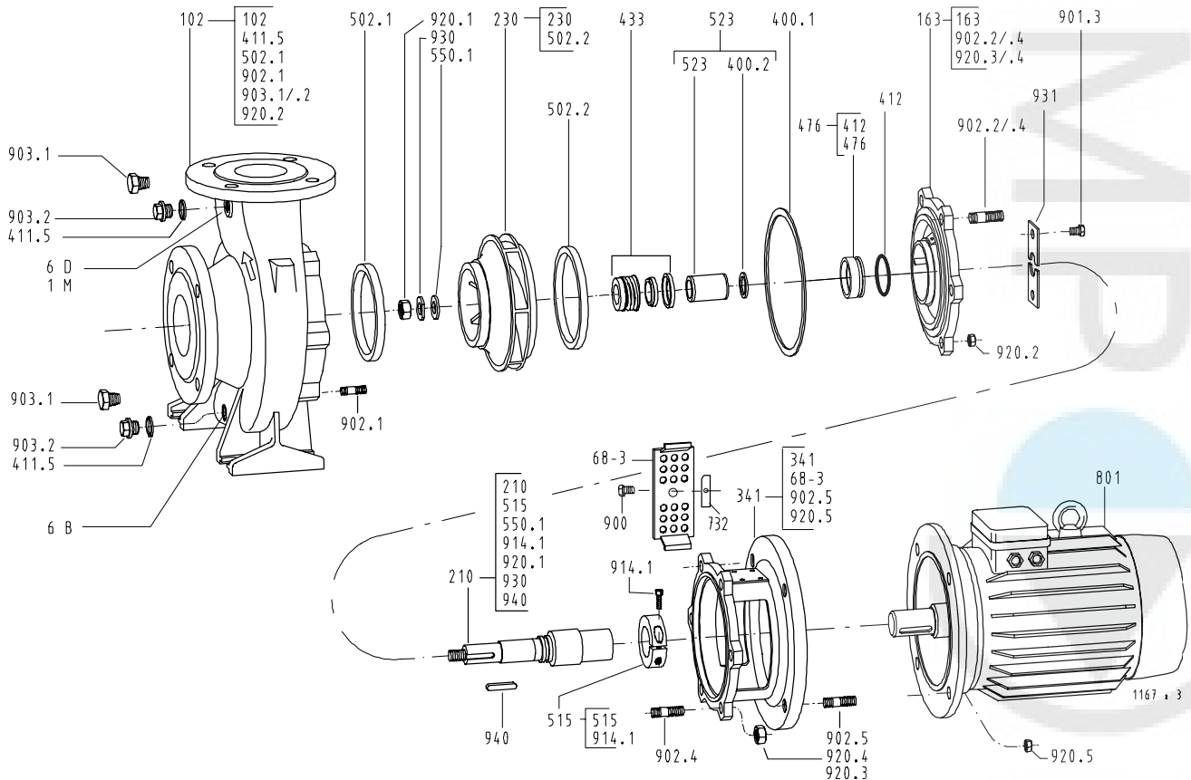
Afbeelding 14: Met genormeerde mechanische asafdichting en aangeschroefd persdeksel
