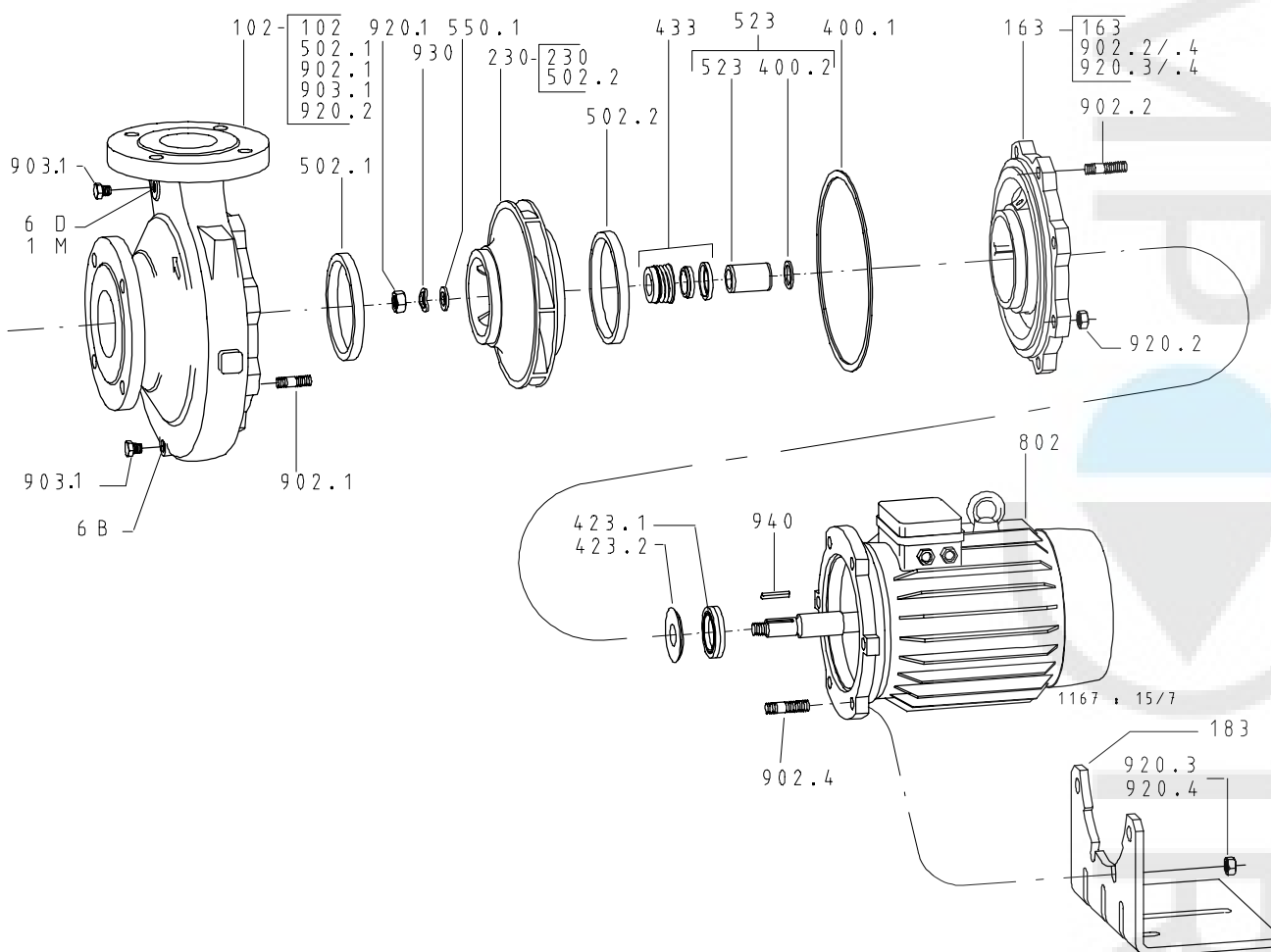
Afbeelding 10: Genormeerde mechanische asafdichting en aangeschroefd persdeksel
