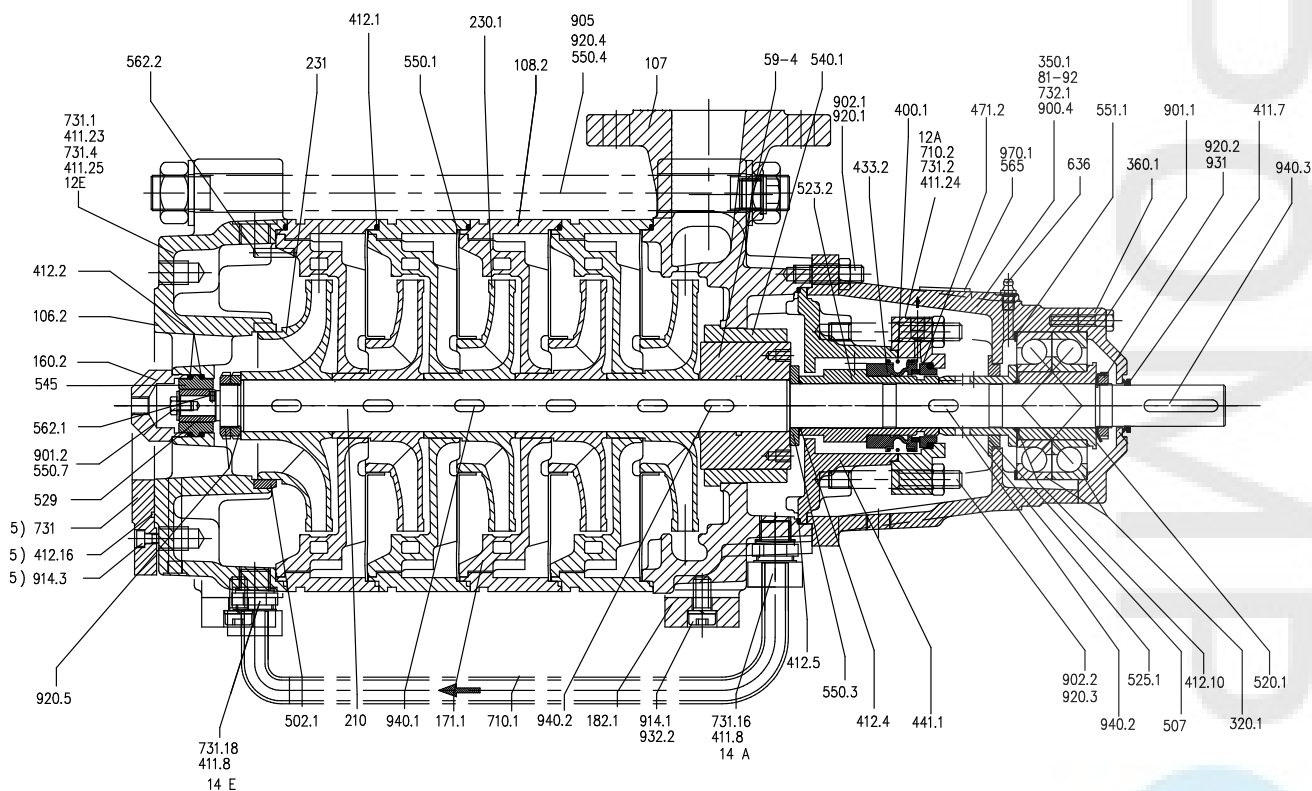
Afb. 54: Multitec-RO - pomp-grootte 50
