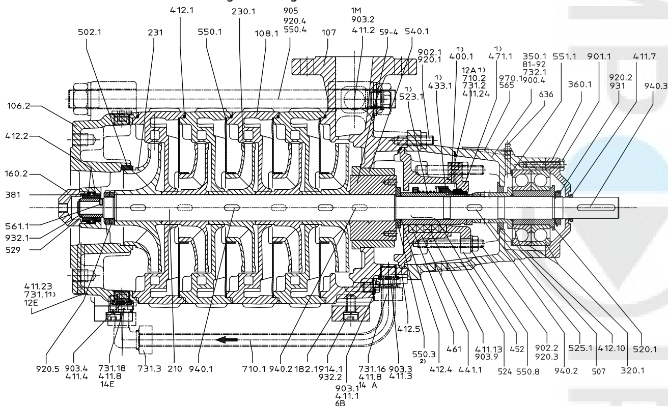
Afb. 51: Multitec - opstellingstype A - pompgrootte 32-50
